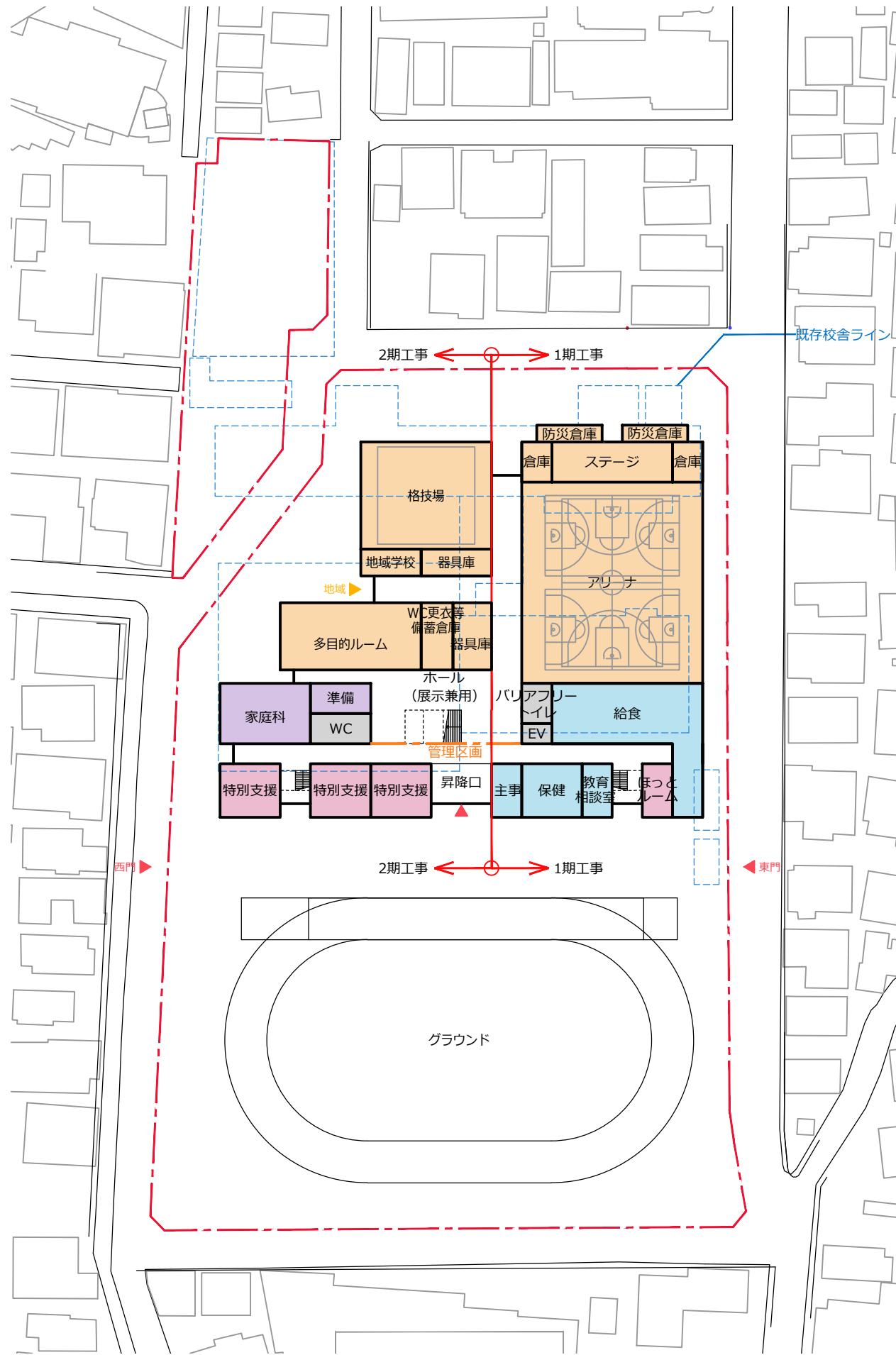
<配置図兼1階>
