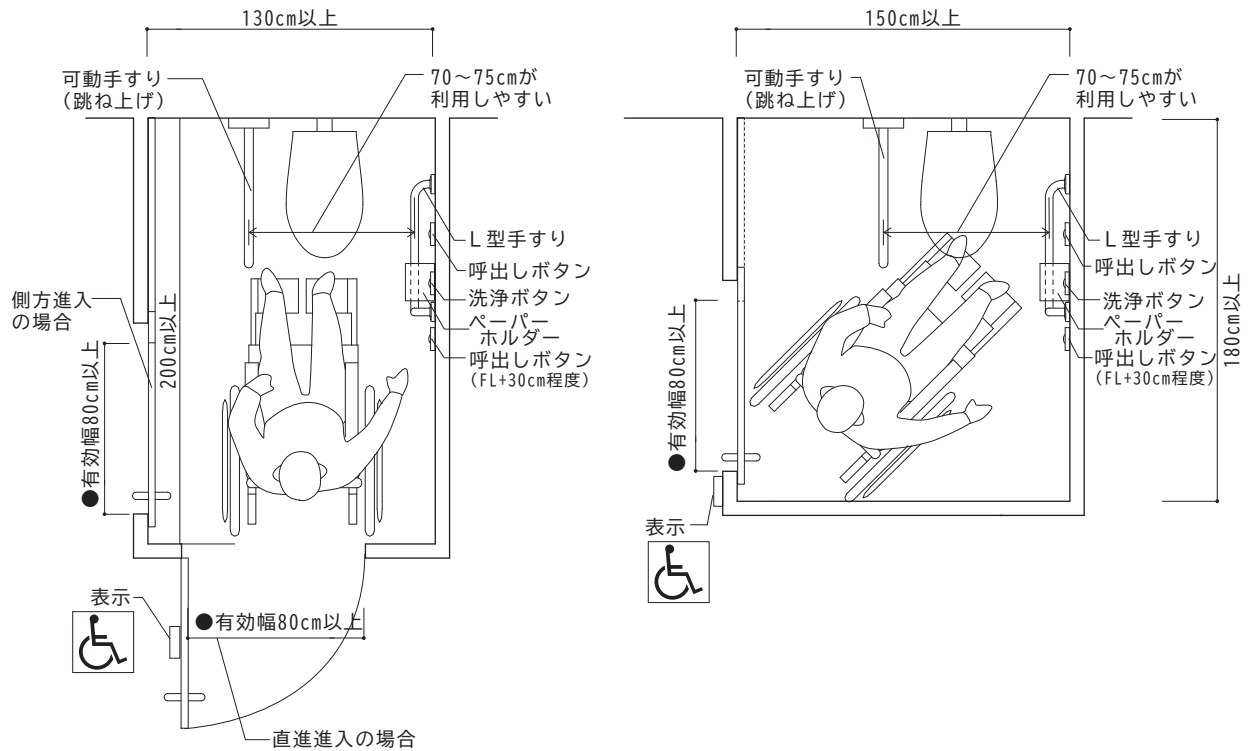
【図2-1】簡易型車椅子使用者用便房の例
