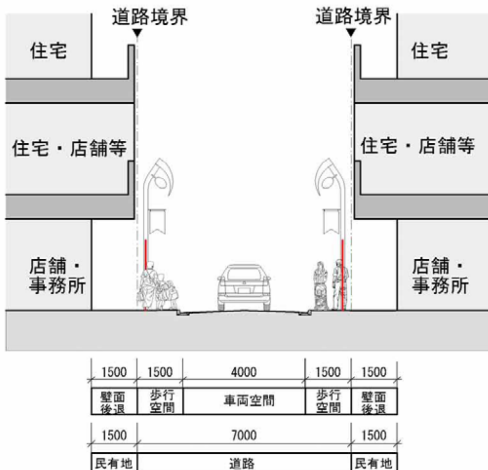
区間B 標準断面図（城山通り以南）
