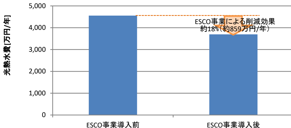
図:光熱水費の令和3年度実績値
