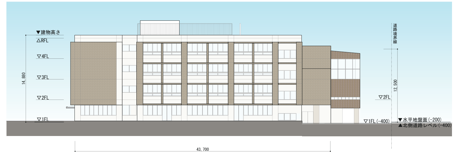
東立面図
