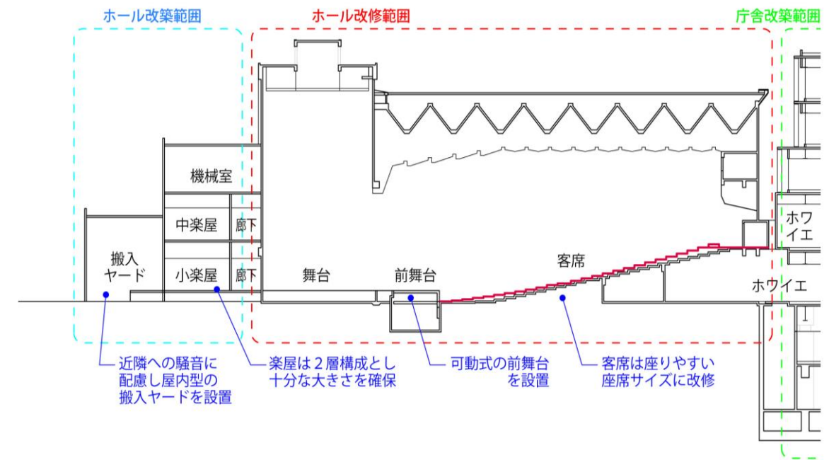
断面図
