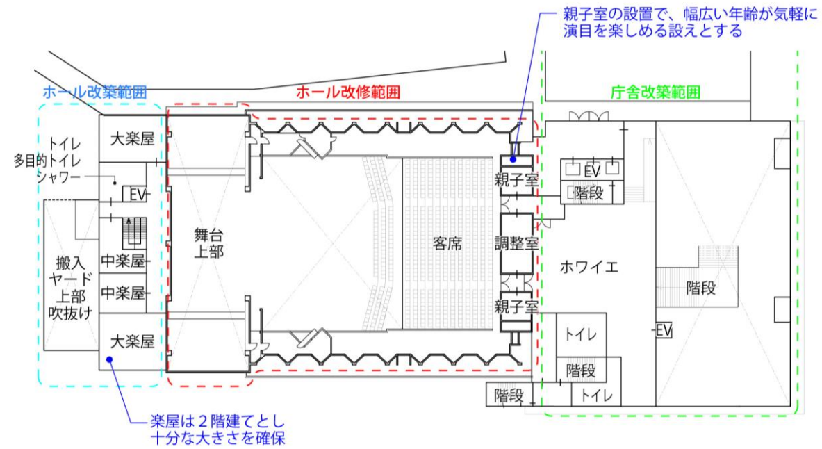
2階平面図
