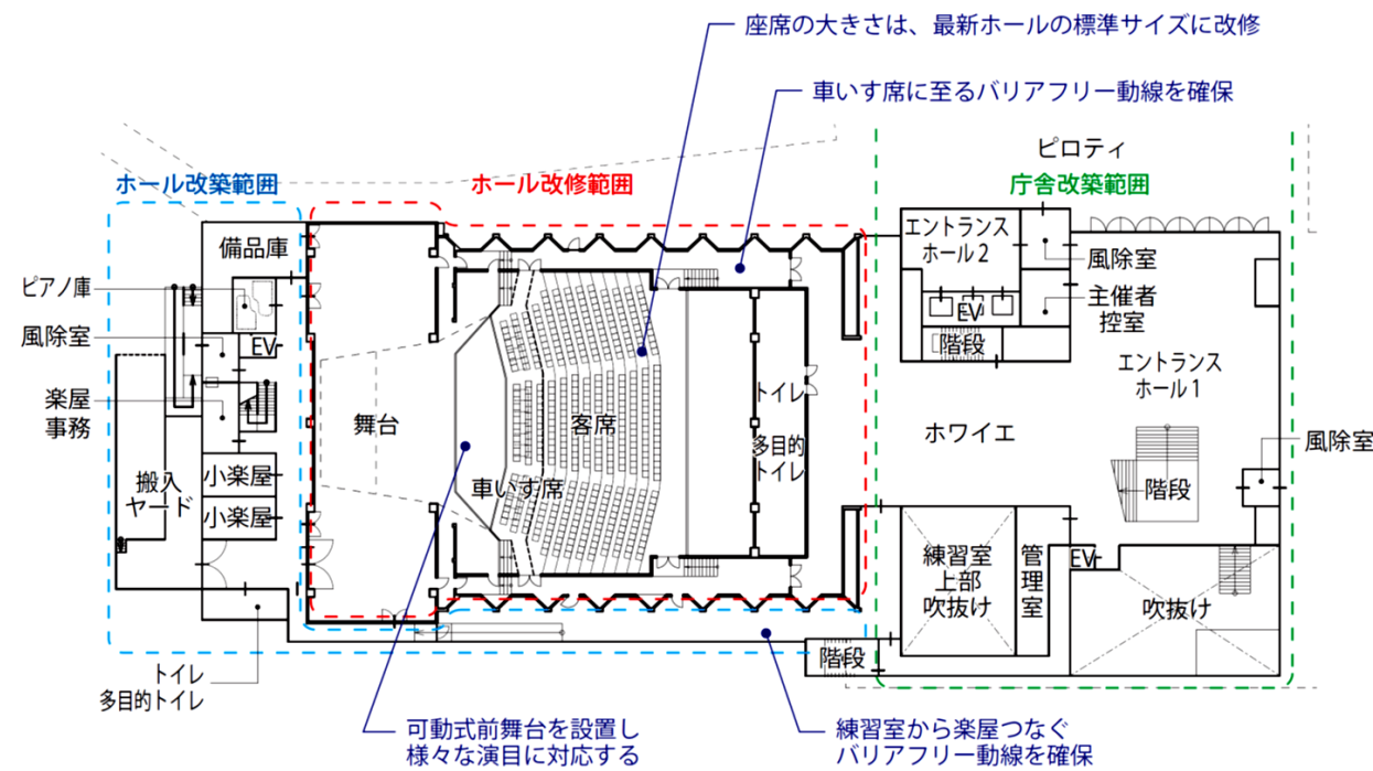
1階平面図
