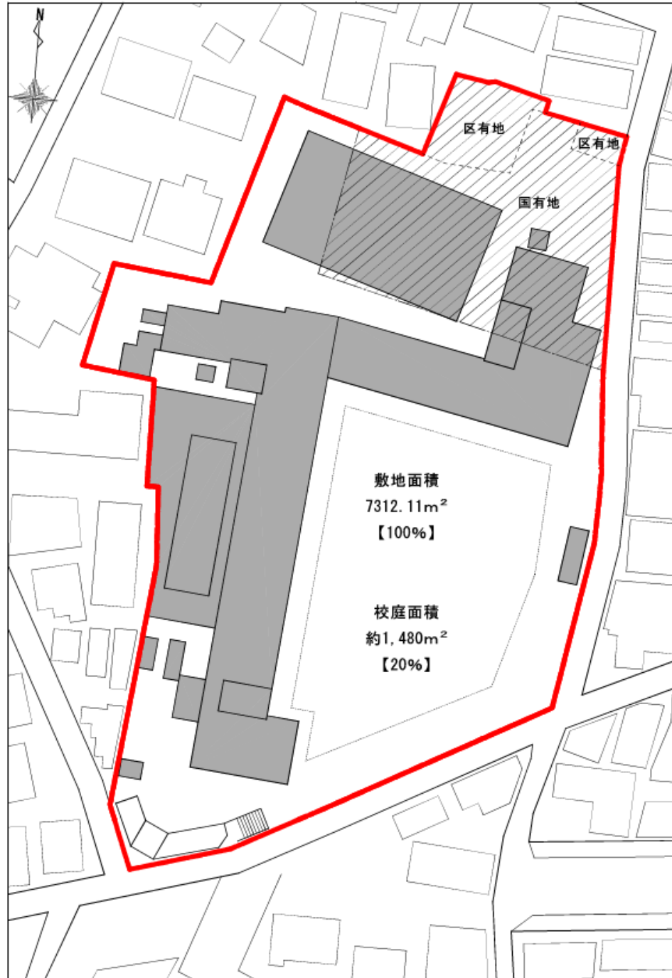
■現況敷地図
