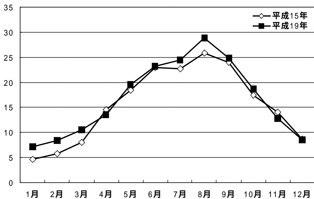
第2図 月次別平均気温 (世田谷観測所)
