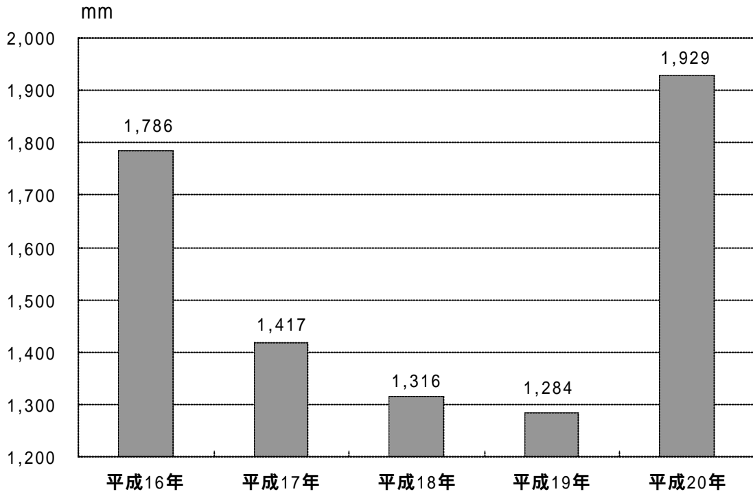
第1図 年間降水量の推移 (世田谷観測所)
