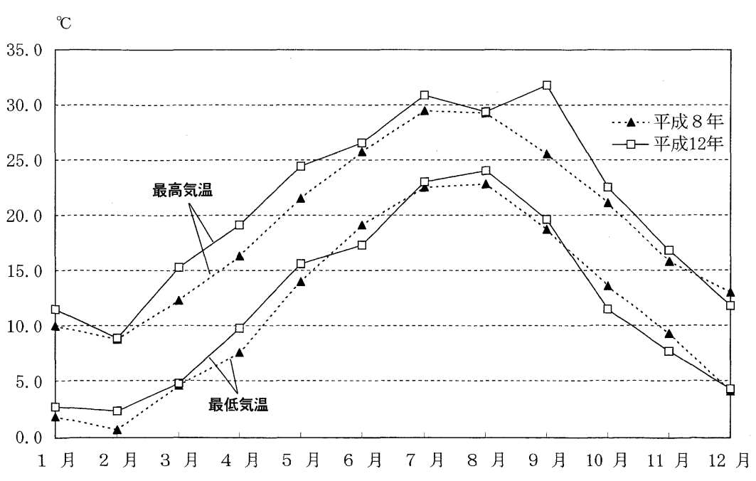
第2図 月次別最高気温と最低気温(世田谷観測所)
