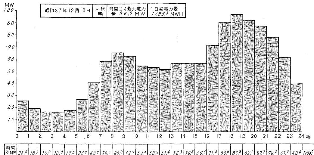
第 1 図 時間別使用電力量
