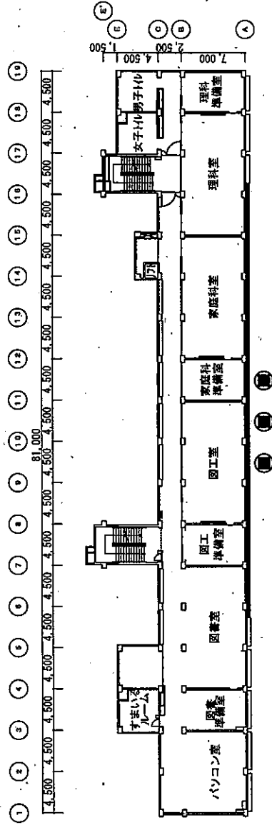
屋上階平面図
