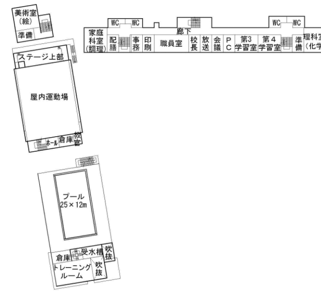
弦巻中学校 2階平面図
