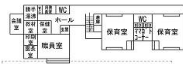
松丘幼稚園 1階平面図
