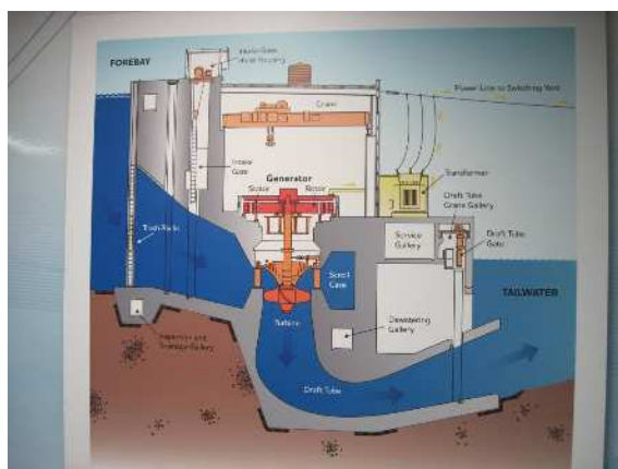
水力発電所断面図
