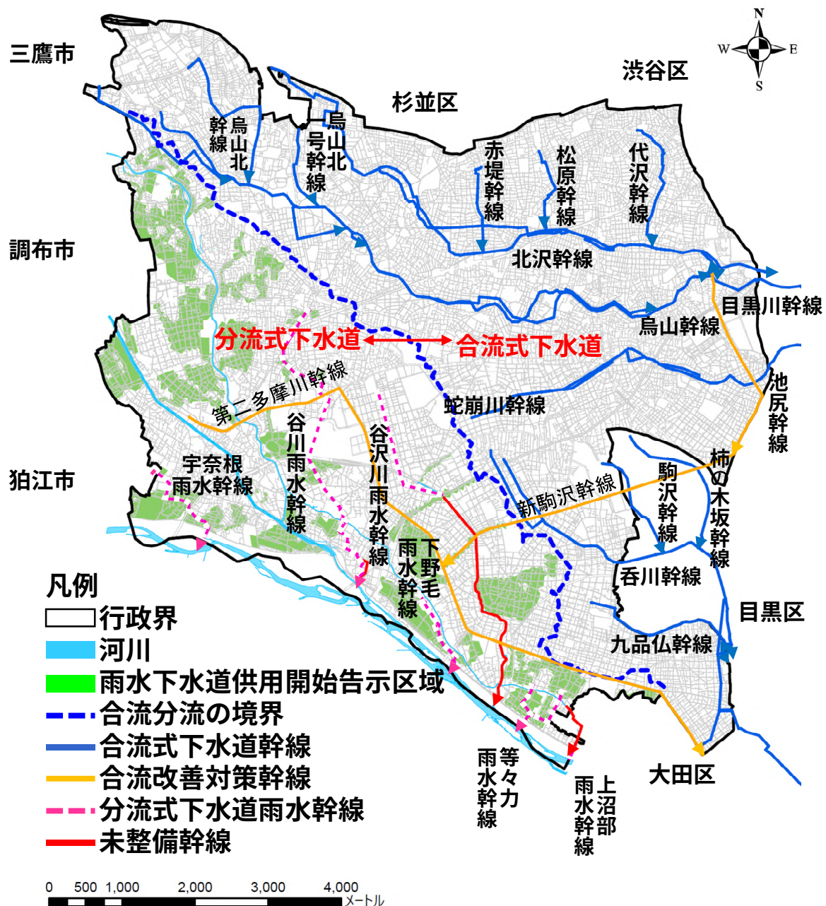
図2.2 下水道（雨を流す幹線）の整備状況図（令和元年7月現在）
