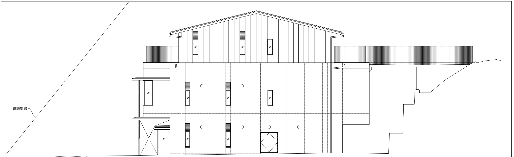
東側立面図
