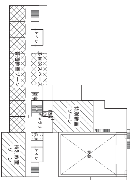
2階平面図
