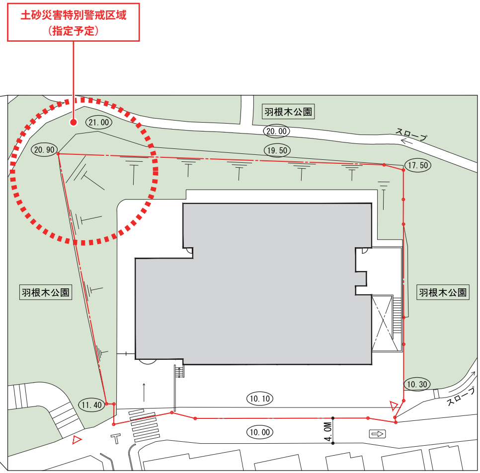
配置図
