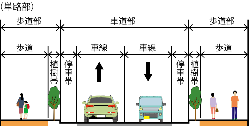
図 3- 3 往復 2 車線道路の評価幅員の横断面構成
