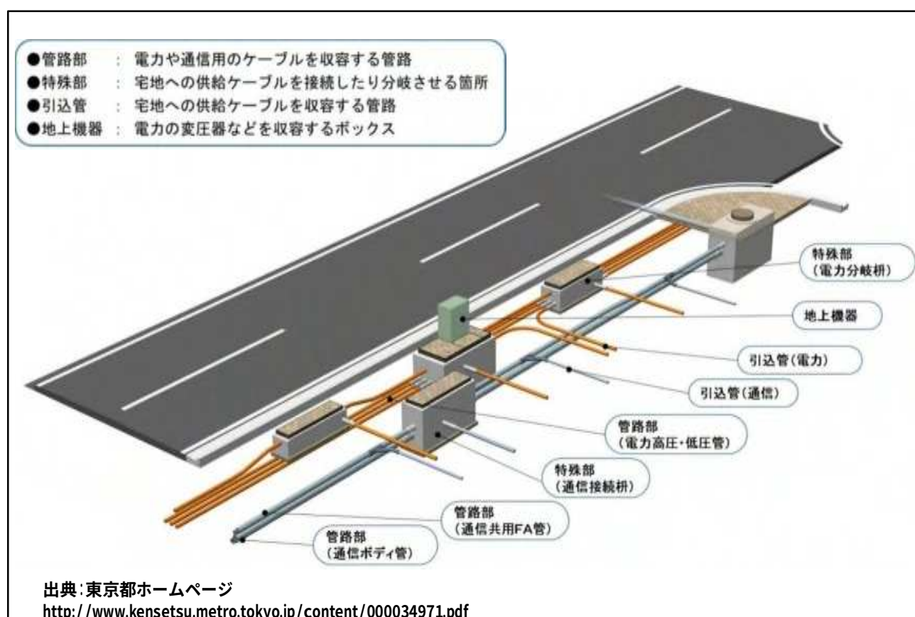
図表 3.2 電線共同溝のイメージ
