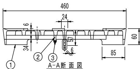
A-A断面図
