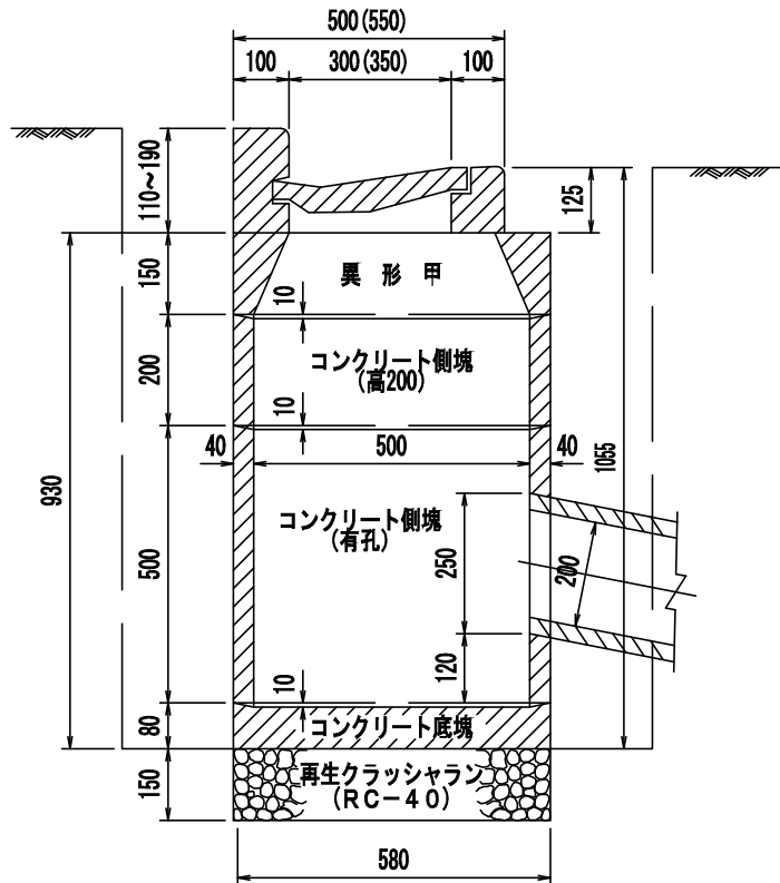
B-B 断面図
