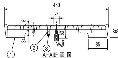
A-A断面図
