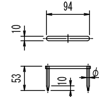
取手詳細図
