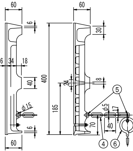
側面図
