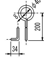
フック詳細図
