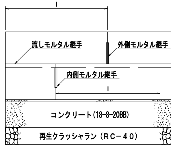
側面図
