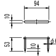
取手詳細図
