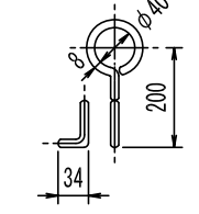
フック詳細図
