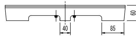
正面図
