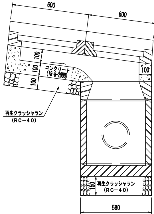
A-A 断面図
