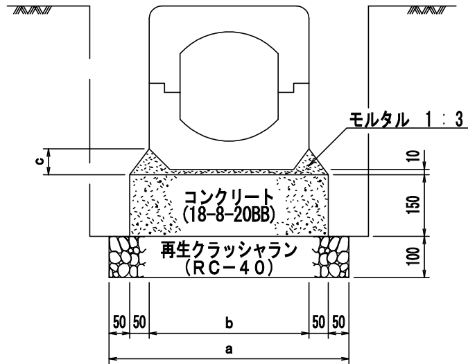
寸法表
