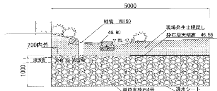
レインガーデン 断面図
