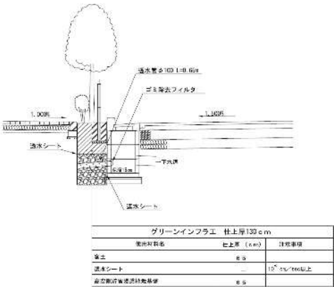
グリーンインフラ工構造図 3/15
