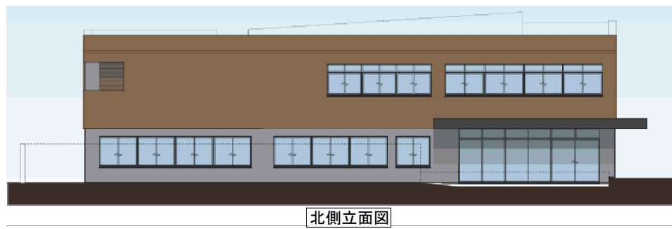
北側立面図
