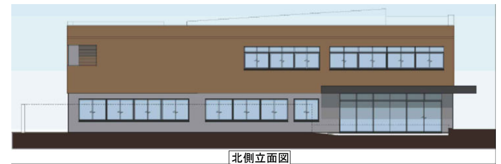
北側立面図
