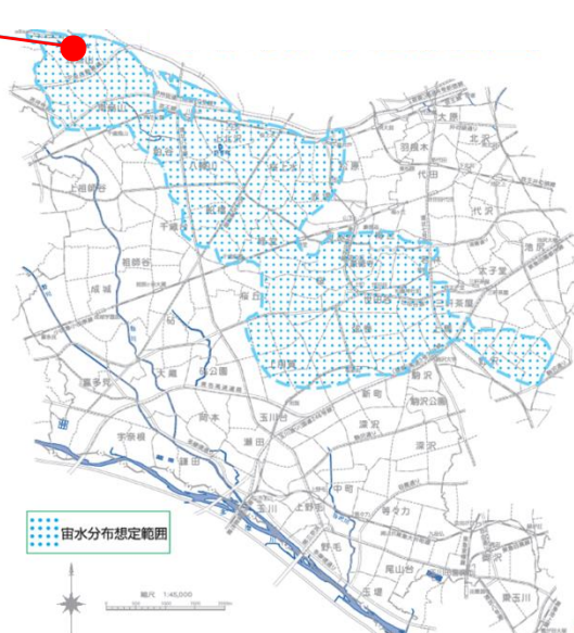
宙水分布想定図 (出典:宙水をご存知ですかパンフレット)
