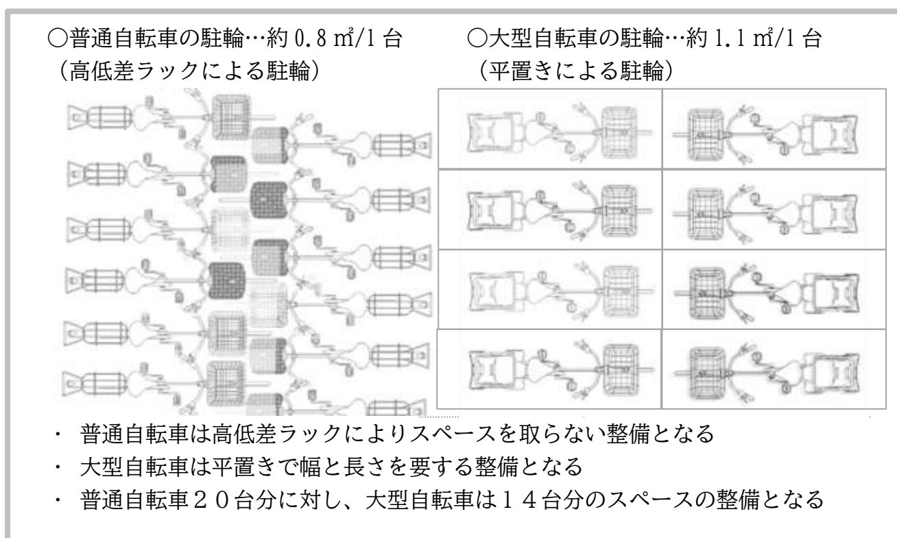
図 29 普通自転車と大型自転車の駐輪スペースの比較（イメージ図）
