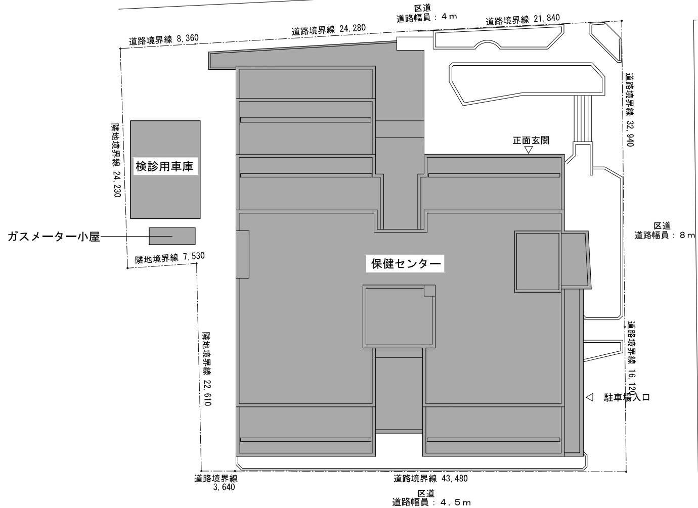
解体建物配置図
