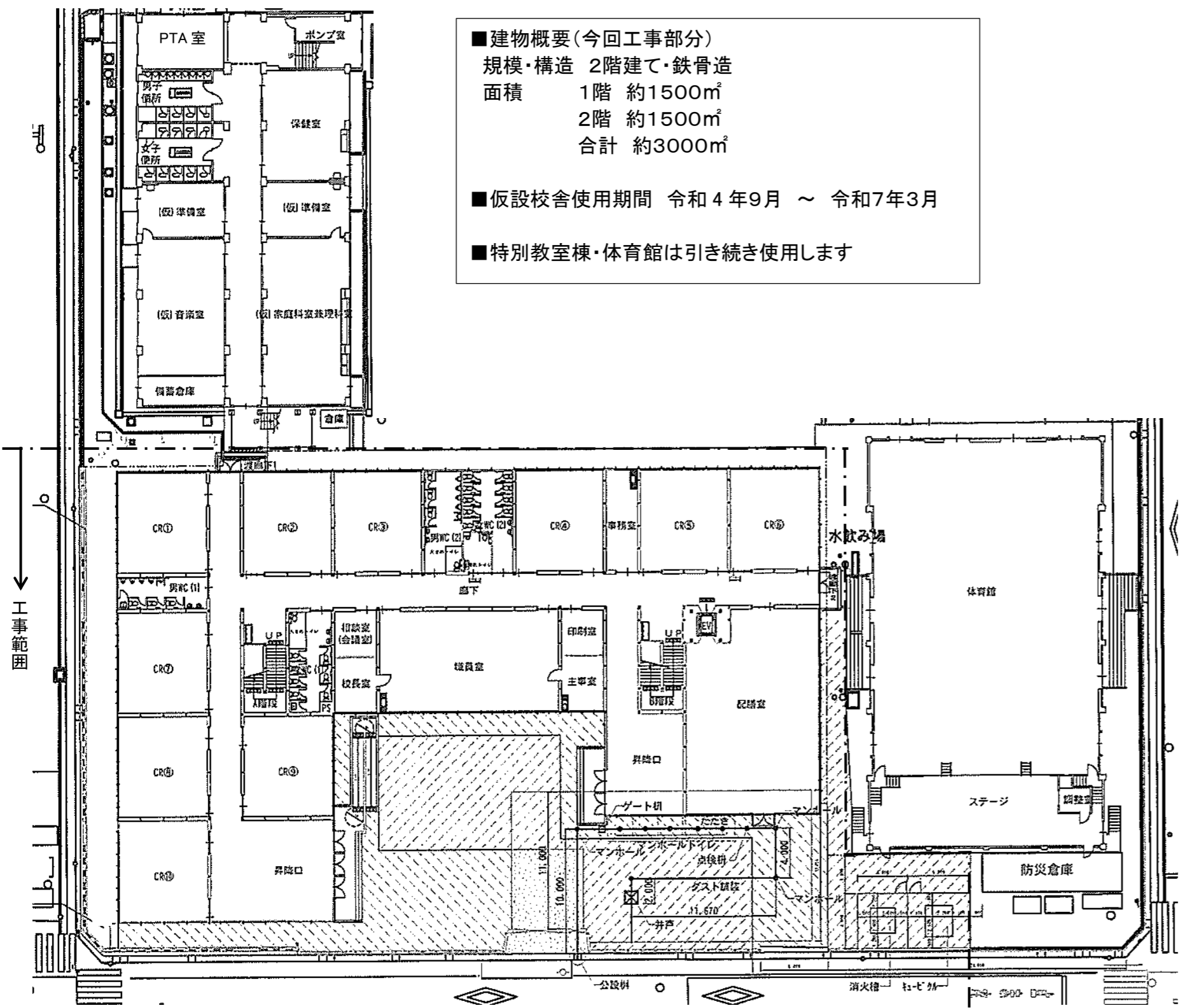
1階・配置平面図
