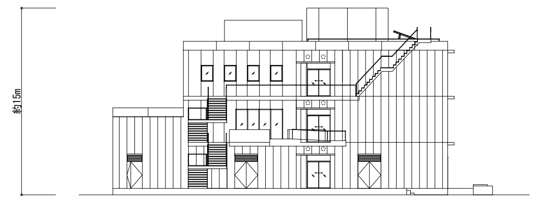
西立面図
