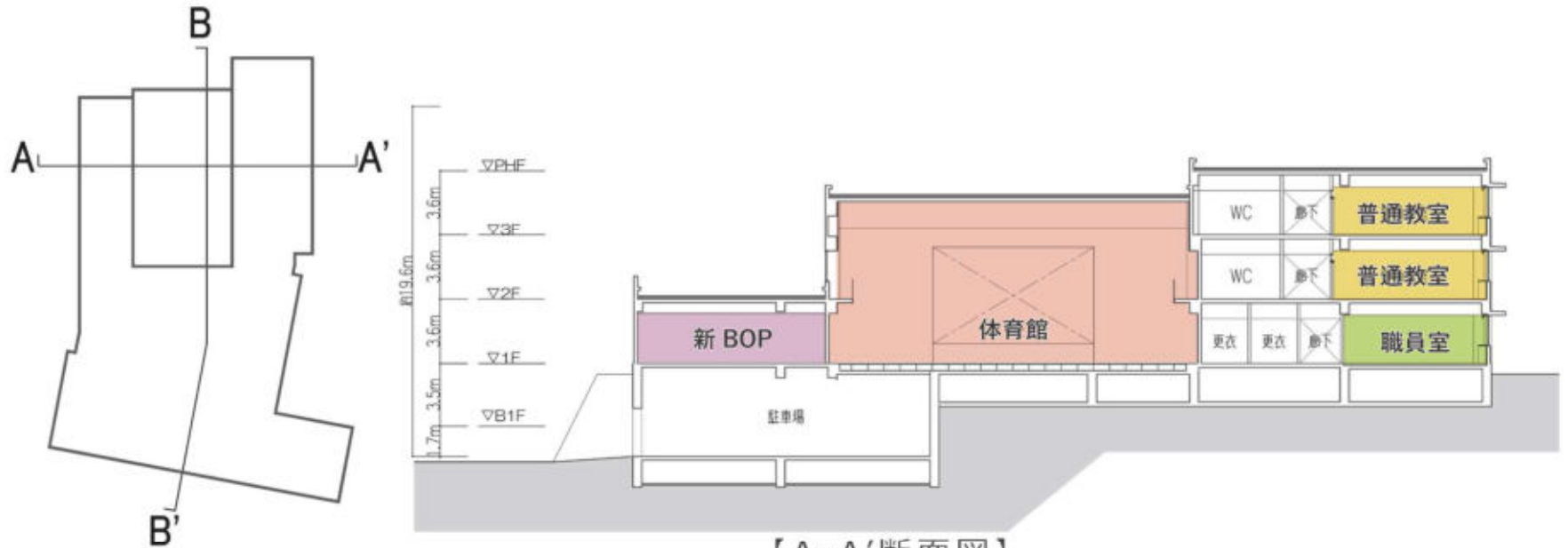
【A-A'断面図】
