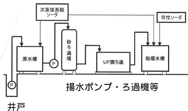
災害対策用井戸（システムイメージ）
