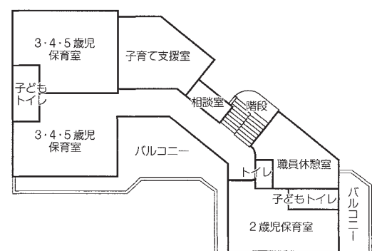
<2階>
