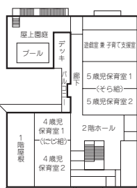
2階平面図
