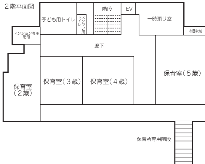
2階平面図
