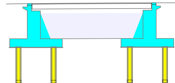
橋台断面図
