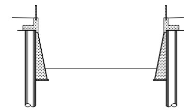
護岸断面図
