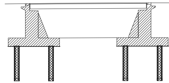
橋台断面図
