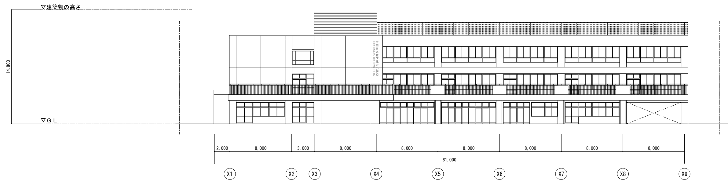
校舎棟 南側立面図
