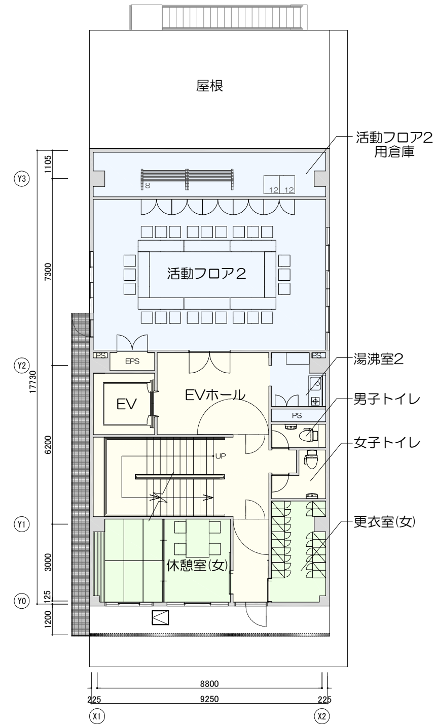
4階平面図
