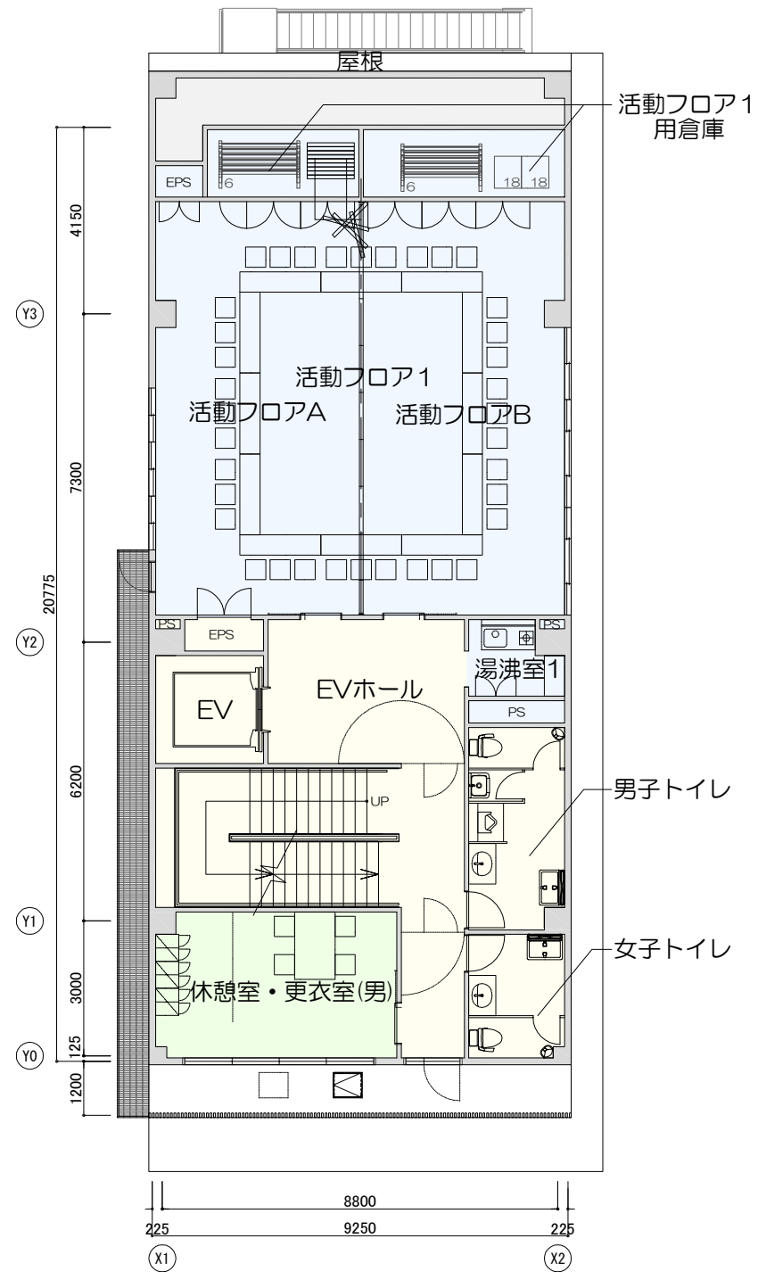
3階平面図
