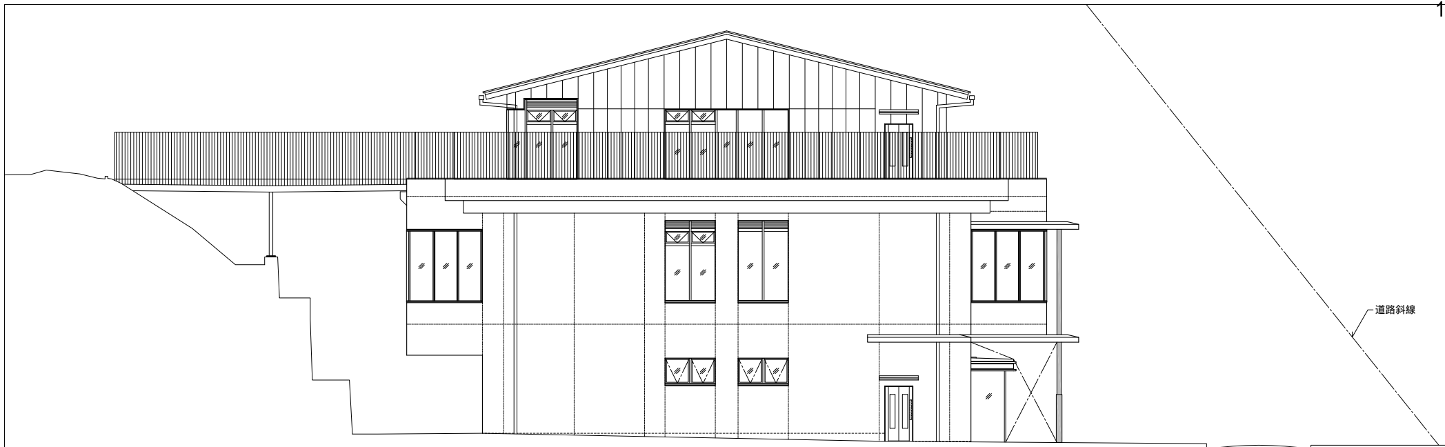
西側立面図
