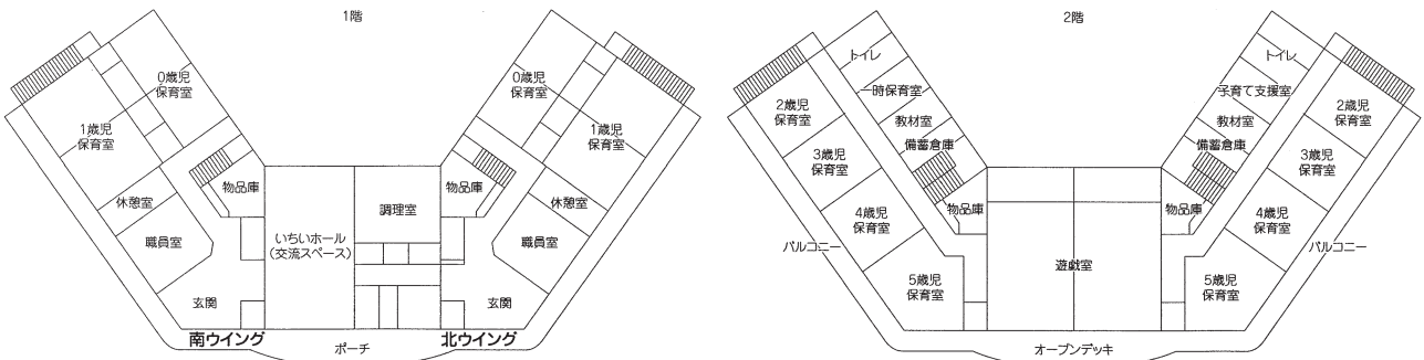
【平面図】
